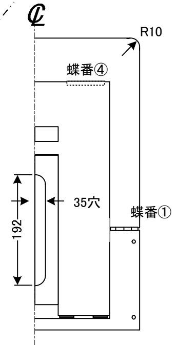
収納時正面図
